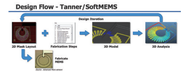
▲ 「微機電開發平台」設計流程 "MEMS Development Platform" design process
